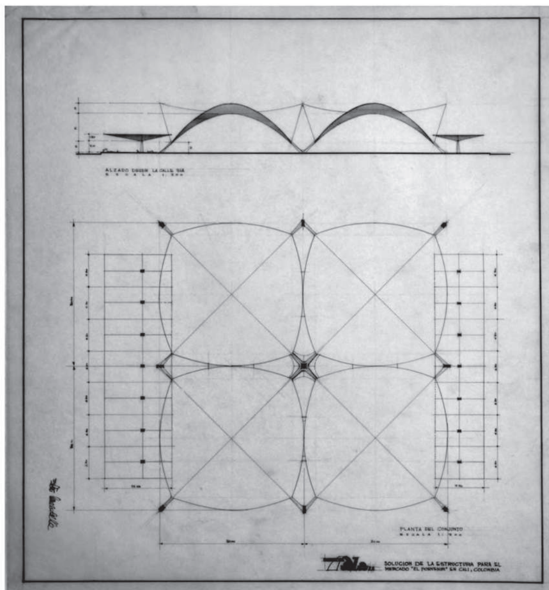
Figura 6. Una de las soluciones de bóvedas elaboradas por Cubiertas Ala Colombia para la Plaza del Mercado El Porvenir en Cali. Félix Candela architectural records and papers, 1950-1984, Avery Architectural & Fine Arts Library, Columbia University.
