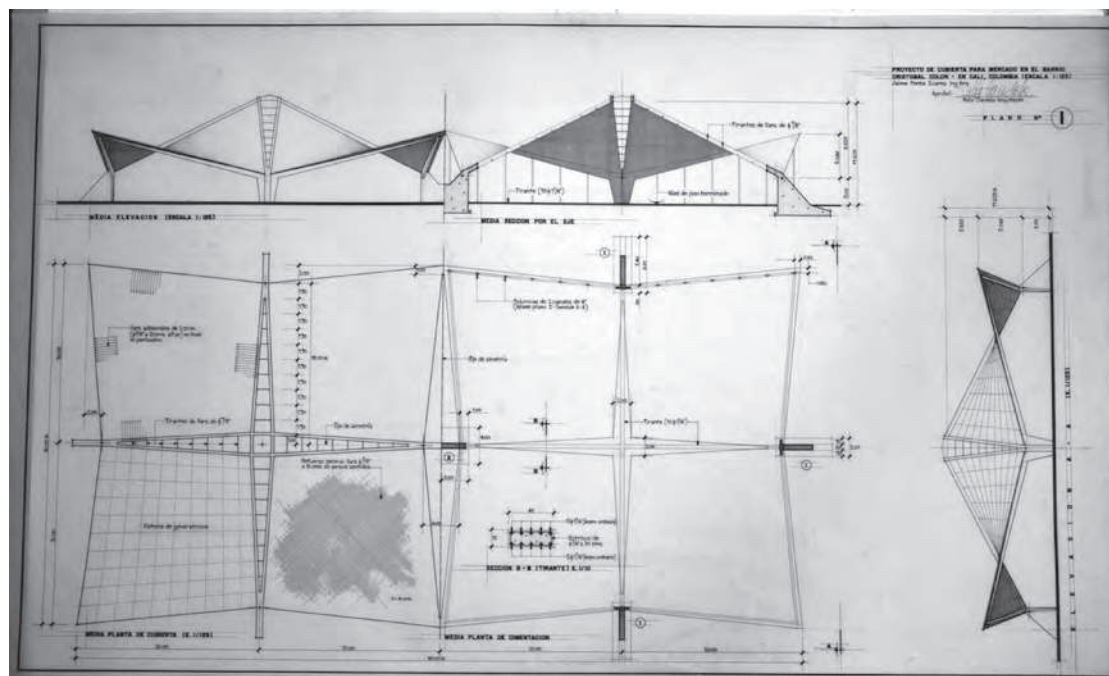
Figura 5. La Plaza del Mercado de Santa Helena (o Colón) en Cali de Cubiertas Ala Colombia. Félix Candela architectural records and papers, 1950-1984, Avery Architectural & Fine Arts Library, Columbia University.
