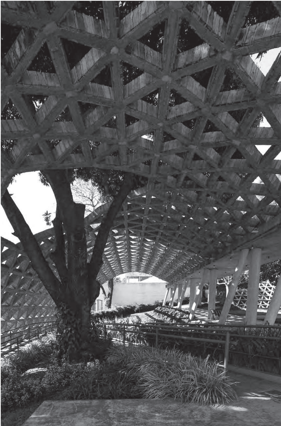
Figura 9 Fundación Teletón, Solano Benítez, Paraguay. Por Federico Cairoli (2010).
