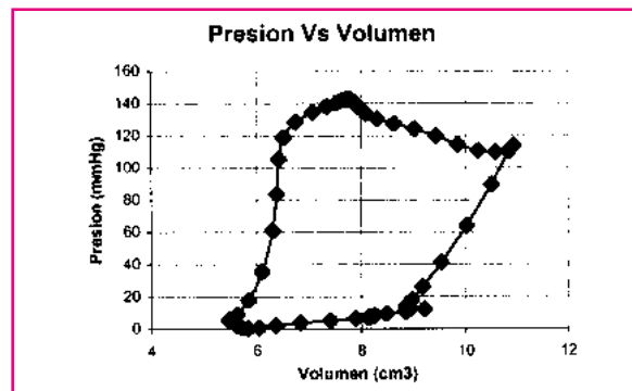
Figura 14. Gráfica Presión Vs Volumen para el caso 1
