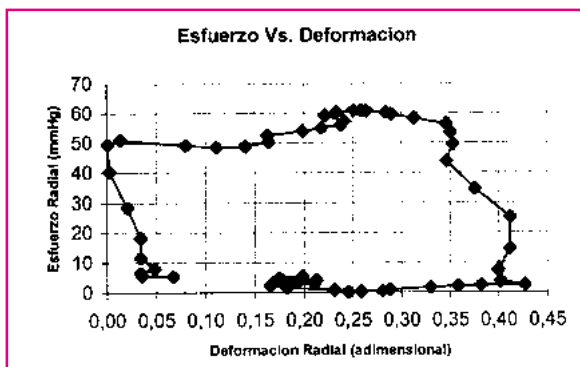
Figura 16. Gráfica Esfuerzo Vs Deformación para el caso 1
