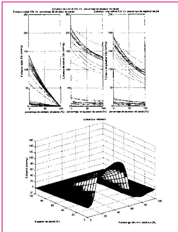
Figura 8. Esfuerzos Principales vs. Espesor de pared Superior: Esfuerzos radial Longitudinal y latitudinal vs espesor de pared, para diferentes presiones (colores). Inferior: Esfuerzo radial vs. Espesor de pared vs. % del ciclo cardiaco
