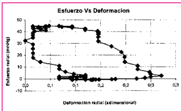
Figura 17. Gráfica Esfuerzo Vs Deformación para el caso 2
