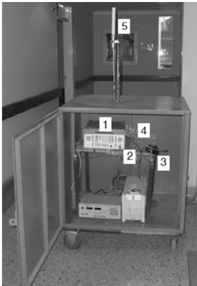
Figura 4. Módulo Transmisor.
