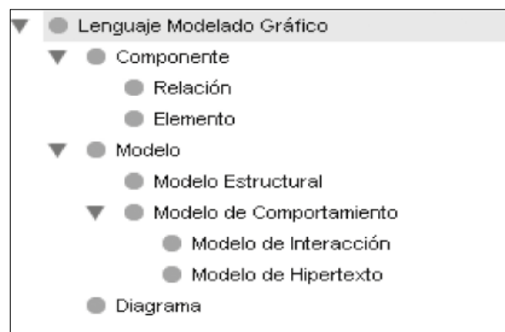
Figura 1. Jerarquía de clases para la ontología propuesta para los lenguajes de modelado gráfico.
